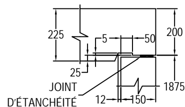
DÉTAIL DU JOINT
