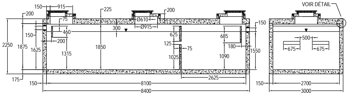
COUPE A
