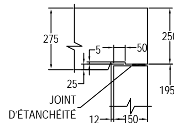
DÉTAIL DU JOINT
