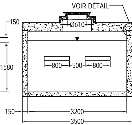
COUPE B
