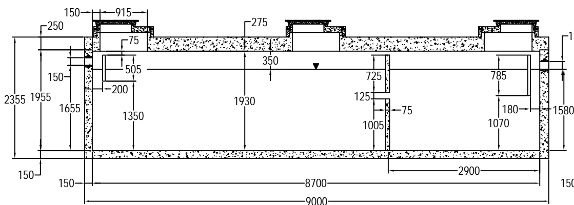
COUPE A
