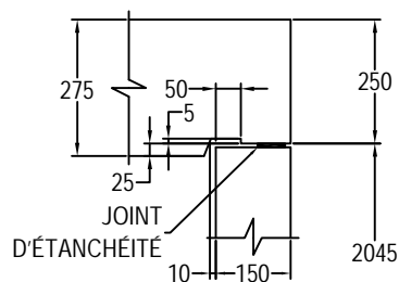
DÉTAIL DU JOINT
