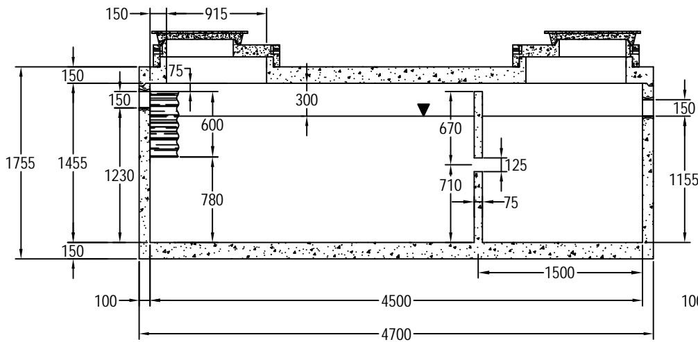
COUPE A
