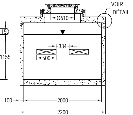
COUPE B
