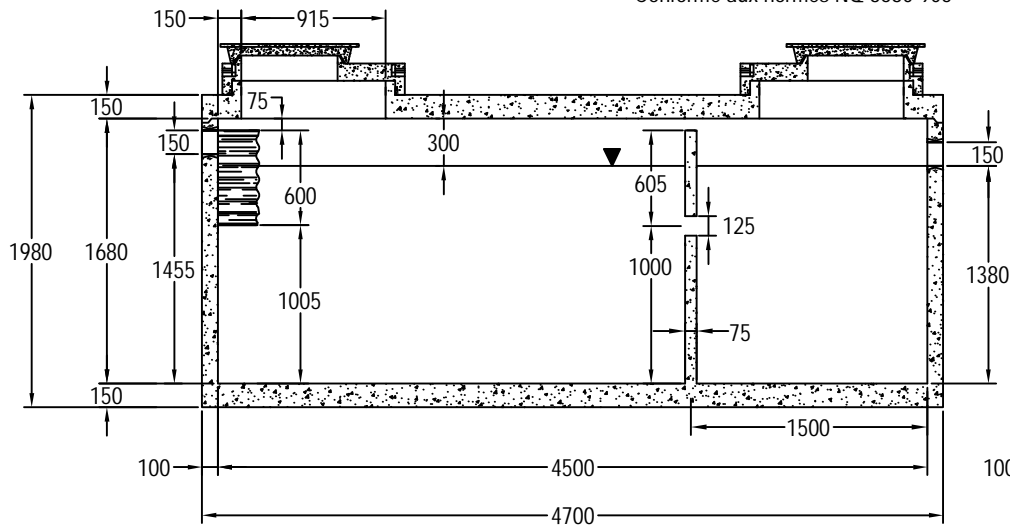
COUPE A
