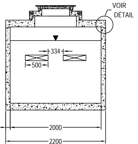
COUPE B
